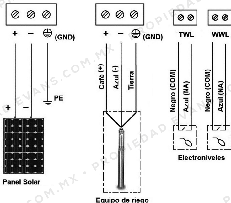
Figura 04. Conexiones en el controlador.
